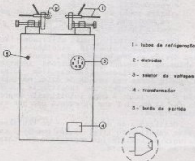
Figura 4. Equipamento de soldagem por resistência elétrica.
