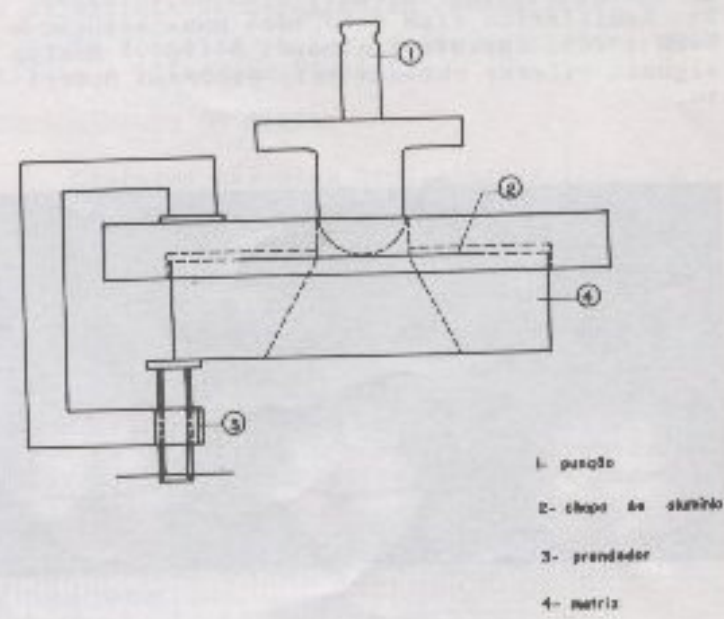
Figura 3. Dispositivo para confecção de hemis- férios.
